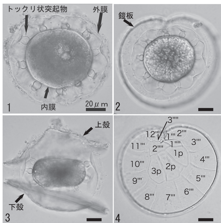
図2. 遺伝子解析に用いた Pyrophacus steinii (Schiller) Wall et Dale の細胞. (1) 標本番号 030702NGt-1, (2)~(4) 標本番号 040623NG-1. (1) シスト ( Tuberculodinium vancampoeae (Rossignol) Wall) の外膜と内膜の間にトックリ状突起物がみられる. (2) 運動性接合子殻内に休眠性接合子 (シスト) が形成されている. (3) 細胞側面観. 扁平な運動性接合子. (4) 運動性接合子下殻の鎧板配列.
