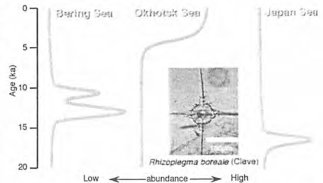
図1. ベーリング海、オホーツク海および日本海における R. boreale の産出頻度を示した模式図。
