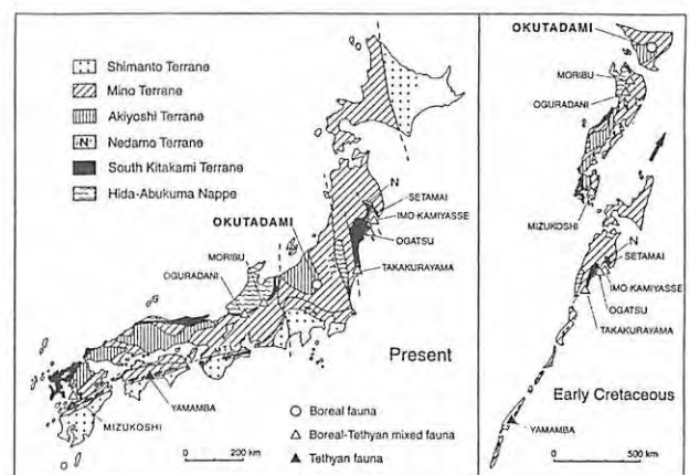
日本のペルム紀腕足類フォーナの地理的分布と前期白亜紀の大規模左横ずれ運動。矢印は地帯群の移動方向を示す。
