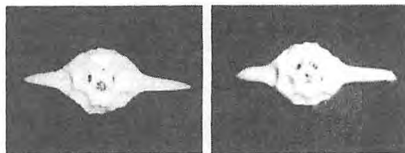
図1 Pantanellium 属放散虫の実体模型。左3号、右4号。
