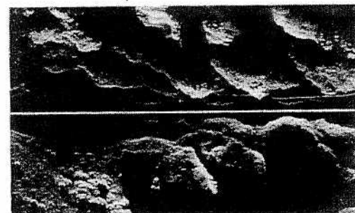
図2 AUVのサイドスキャン(500kHz)で捉えたサンゴ礁の窪地に堆積した泥
