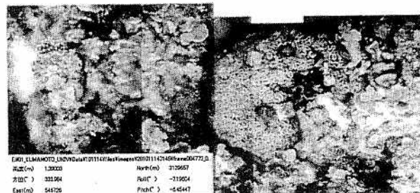
図1 AUVのCCDカメラ(3枚/秒)で撮影されたサンゴの表面
